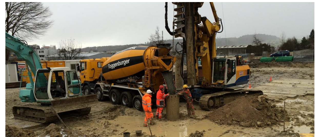
Erstellen der Pfahlfundation
